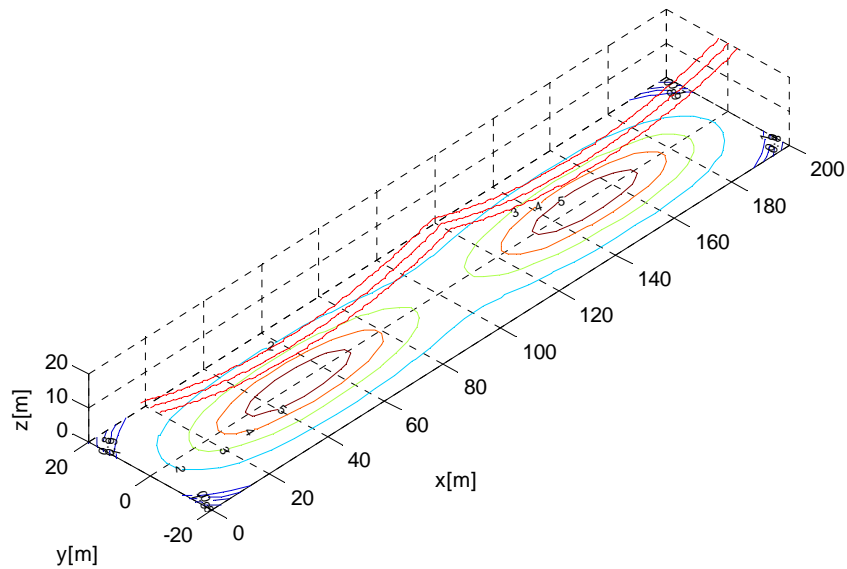
Curve isocampo di Induzione Magnetica B[ \mu T]
