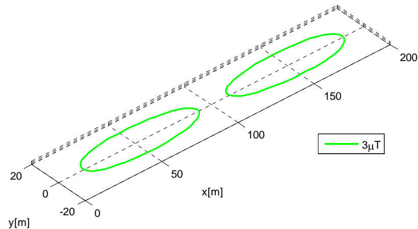
Isocurve di induzione magnetica B=3 \mu T - B=10 \mu T - B=100 \mu T
