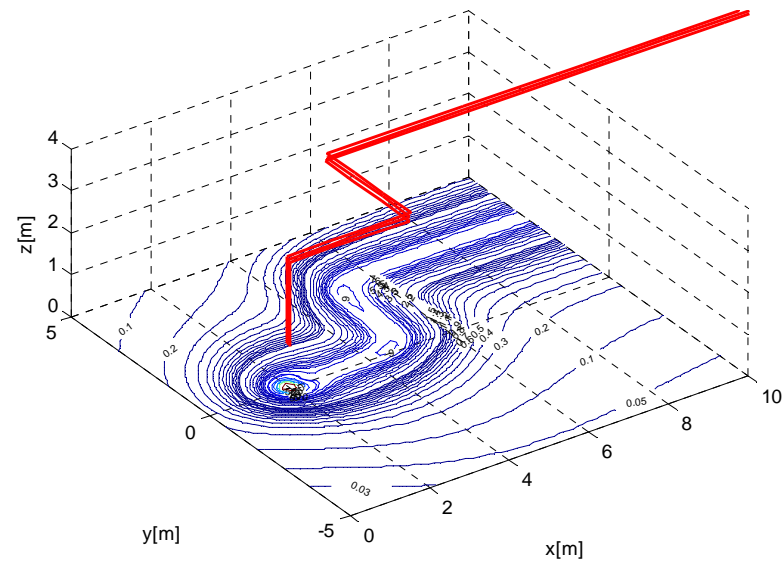
Curve isocampo di Induzione Magnetica B[ \mu T]
