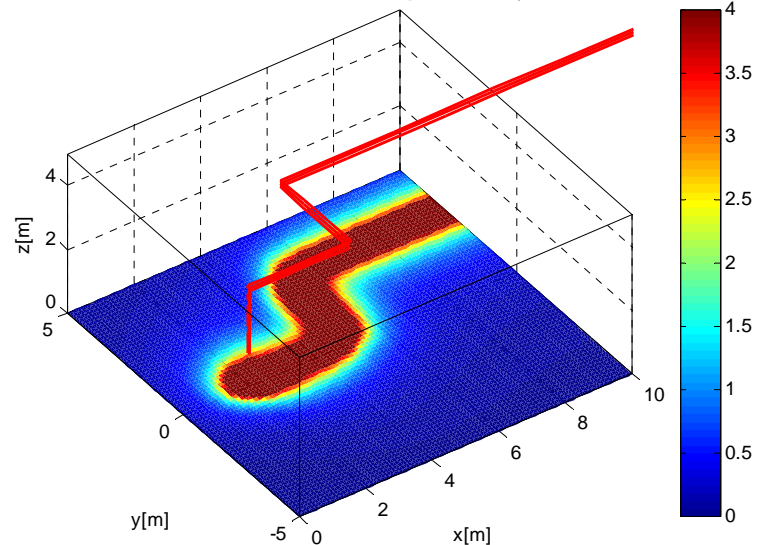
Mapa di induzione magnetica B[ \mu T]
