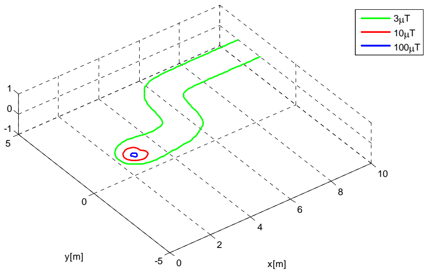
Curve isocampo di Induzione Magnetica B=3 \mu T - B=10 \mu T - B=100 \mu T
